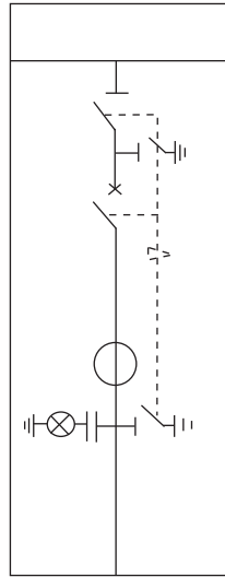
Kescilli Giriş/Çıkış Hücresi (SF6 Gazlı Ayırıcılı)
