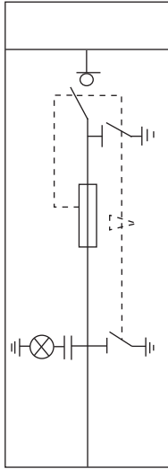
Yük Ayırıcısı + Sigorta Birleşiği Transformatör Koruma Hücresi
