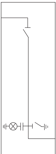
Yandan Çıkışlı Ayırıcılı Bara Bölme Hücresi (SF6 Gazlı Ayırıcı)
