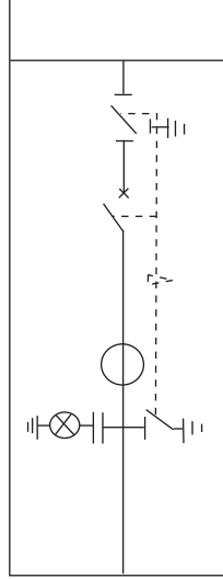
Kescilli Giriş/Çıkış Hücresi (Döner Ayırıcılı)
