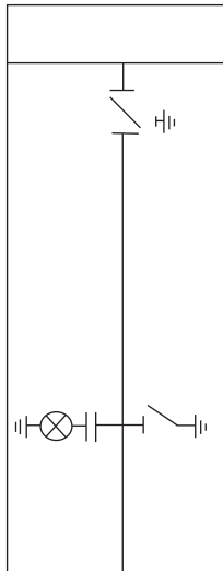
Ayırıcılı Giriş/Çıkış Hücresi (Döner Ayırıcılı)
