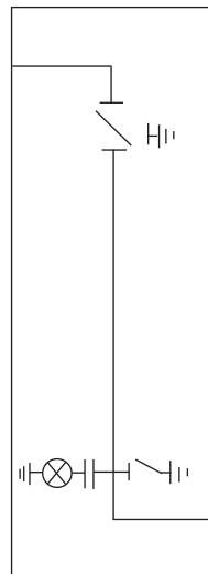
Yandan Çıkışlı Ayırıcılı Bara Bölme Hücresi (Döner Ayırıcı)
