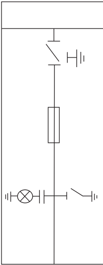
Ayırıcısı + Sigorta Transformatör Koruma Hücresi (Döner Ayırıcılı)
