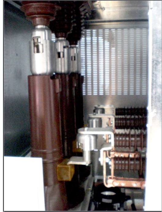
KESİCİ ana devreye BAĞLI
